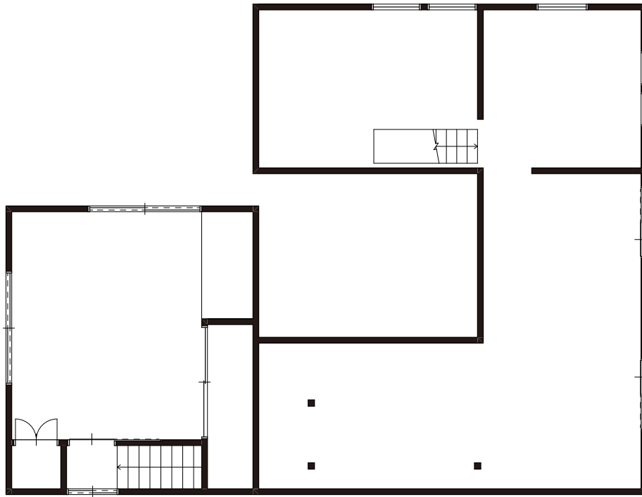
吉田家2階平面図 S=1/100
